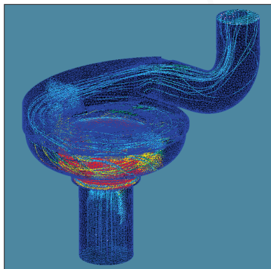
CFD (Вычислительная гидродинамика) анализ полусевого потока гидравлических частей.
