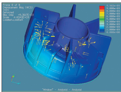
GEM (Геометрические элементы моделирования) анализ спиральной кожура
